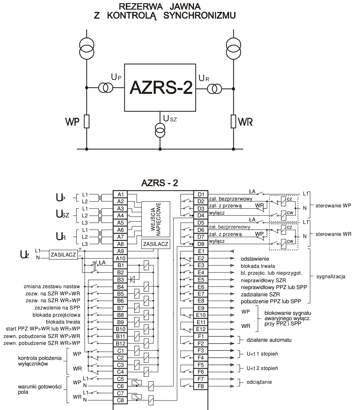
Rys. 7.2.3. Schemat połączeń automatu AZRS-2 zasilanego napięciem pomocniczym przemiennym.
