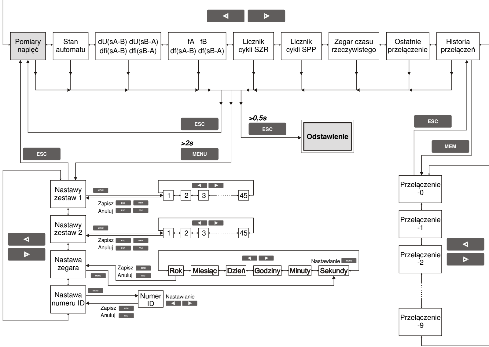
Rys. 8.3. Struktura menu.
