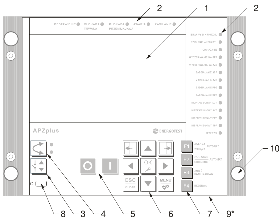
rys. 6 Opis elementów na panelu sterowania.
