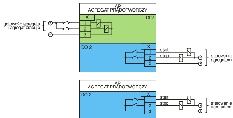
Rys. 39. Przykładowe schematy podłączenia agregatu
