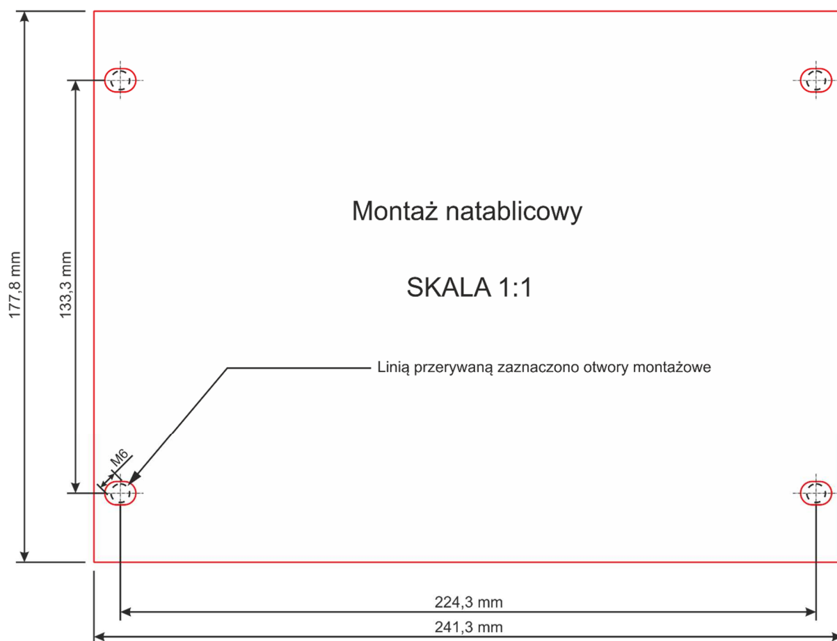
rys. 52 Montaż natablicowy.
