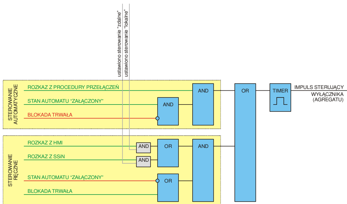
Rys. 43 Sterowanie wyłącznikami (agregatem)
