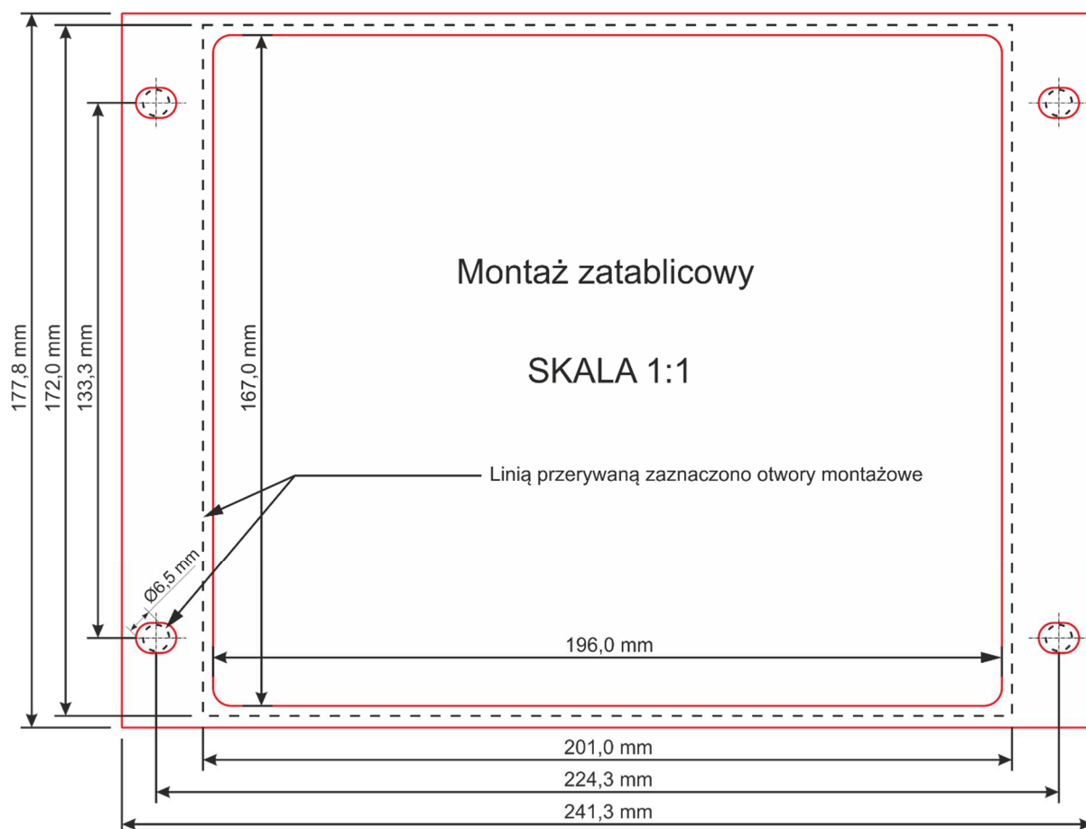
rys. 51 Montaż zatablicowy.
