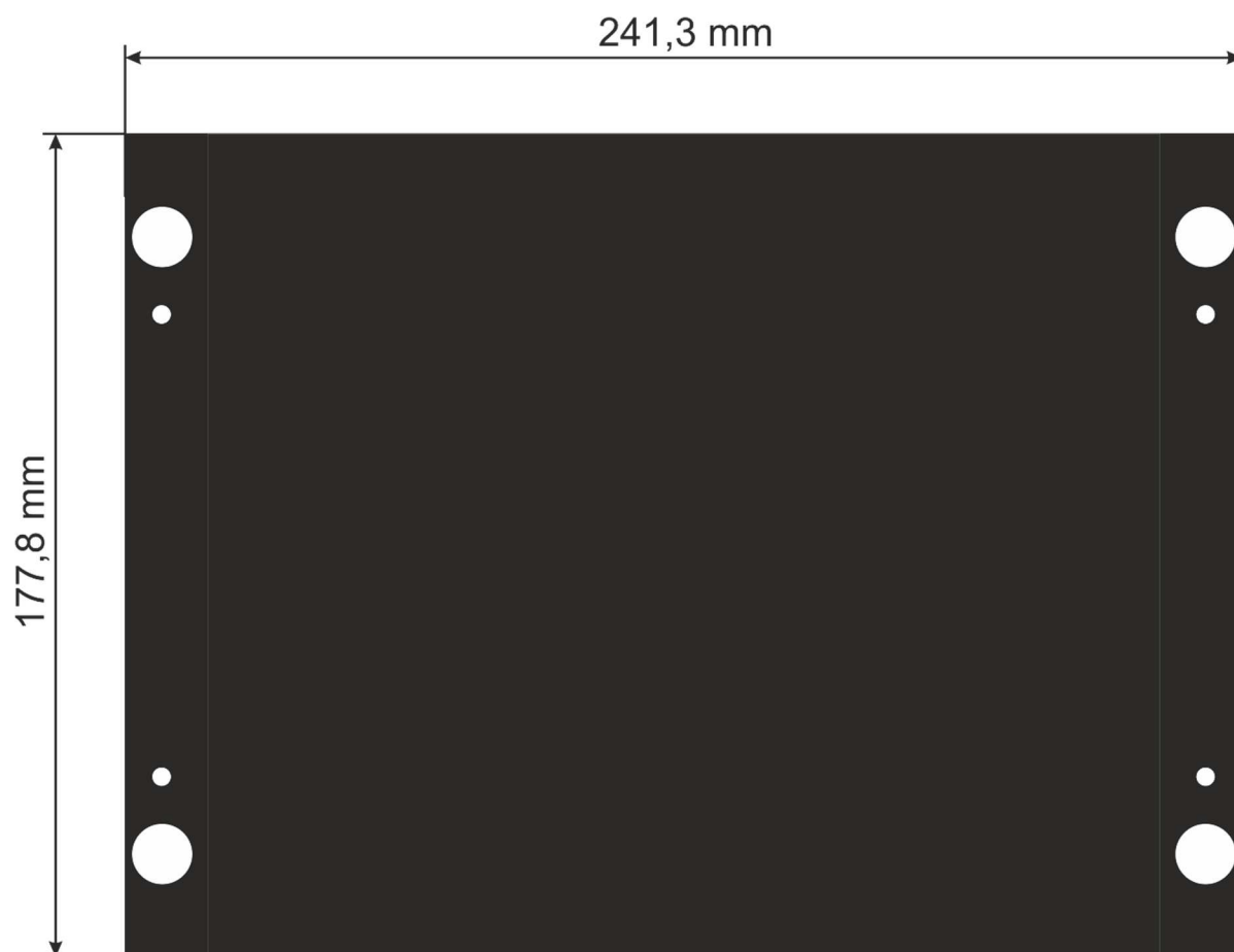
rys.53 Widok tylnej płyty panelu HMI.
