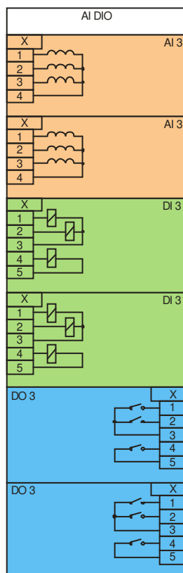
rys. 2. Karta pomiarowa i wejść/wyjść dwustanowych – AI,DIO.
