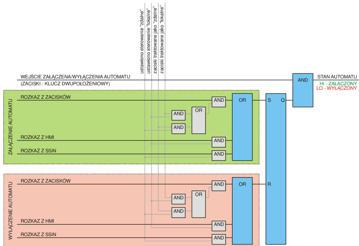
Rys. 40 Sterowanie załączaniem i wyłączaniem automatu
